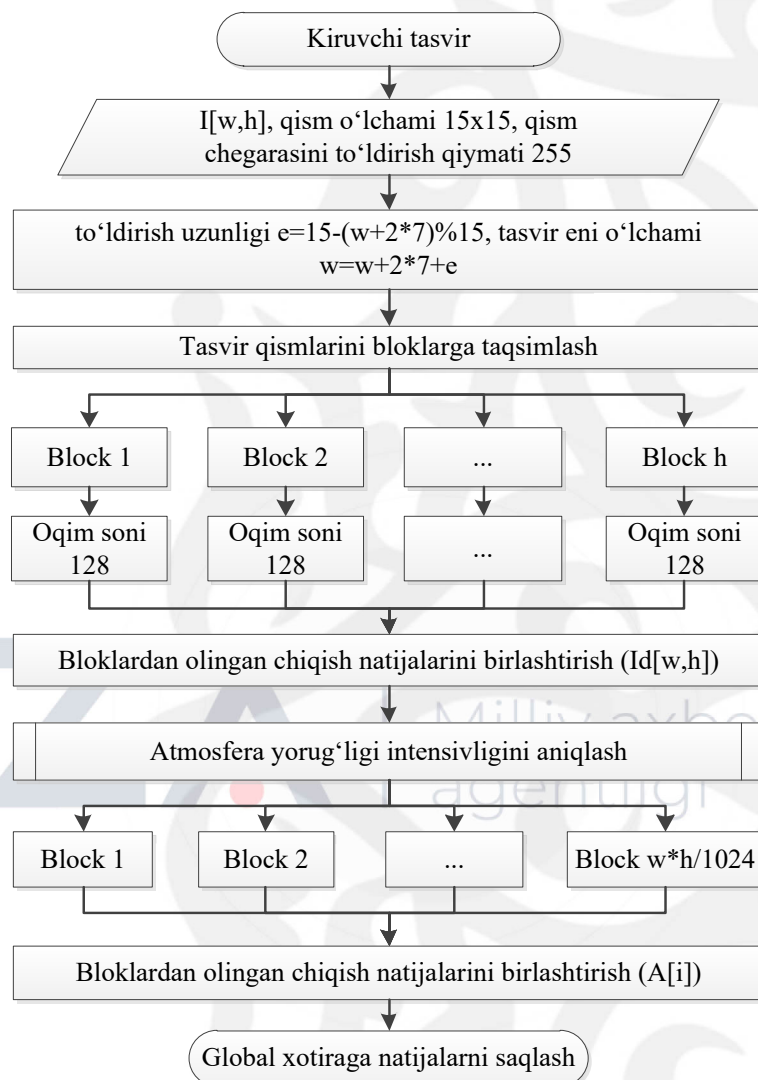
3-rasm. Parallel minimum filtrlash algoritmining blok sxemasi.
