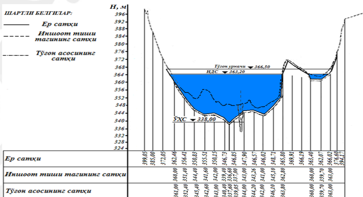
2-расм. Оқтепа сув омборининг 2-навбати тугатилгандан сўнгги ўқи бўйлаб бўйлама кесими.
